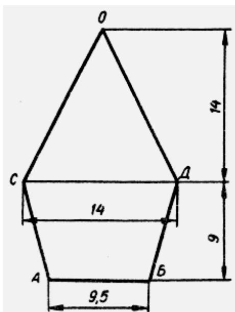
Рис. 6. Креслення клина берета
