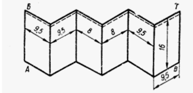
Рис. 3. Креслення спортивної шапочки
