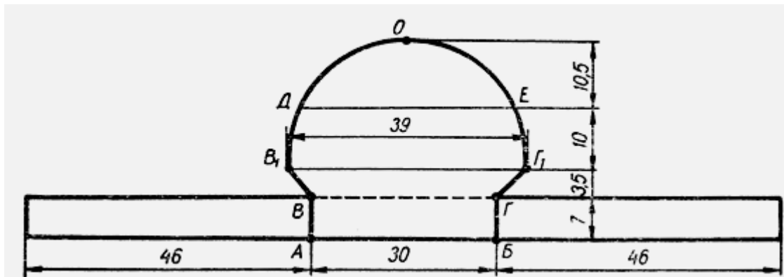
Рис. 5. Креслення шапочки “Українка”
